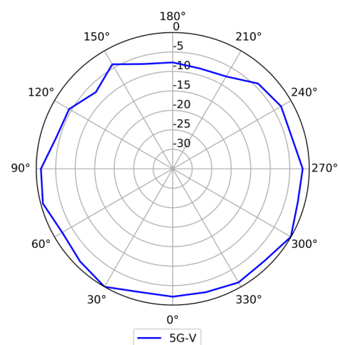
5GHz (Vertical)
