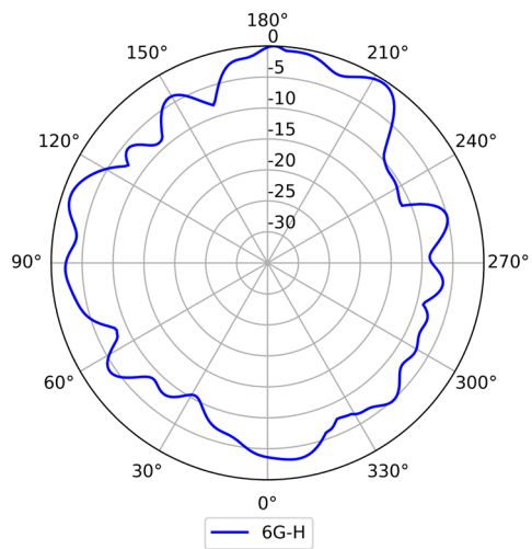
6GHz (Horizontal)
