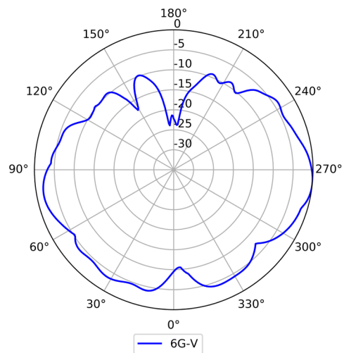
6GHz (Vertical)
